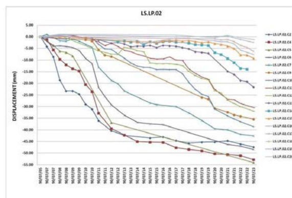
شکل (۷): نشست‌های ثبت شده در محدوده خیابان هلال احمر و کانال رباط کریم [۴]
