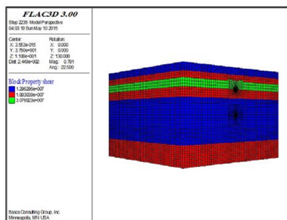
شکل (۵): موقعیت و اعمال پوشش بتنی کانال رباط کریم در مدل
