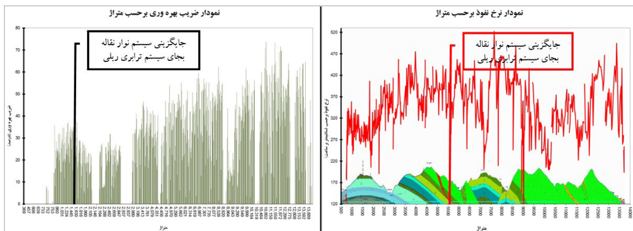
شکل (۱۱): متوسط ضریب بهره‌وری روزانه و نرخ نفوذ در هر کورس حفاری در پروژه تونل بلند زاگرس
