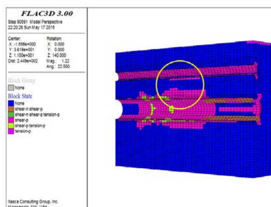
شکل (۱۰): زون پلاستیک ایجاد شده در محدوده کانال رباط کریم در مدل
