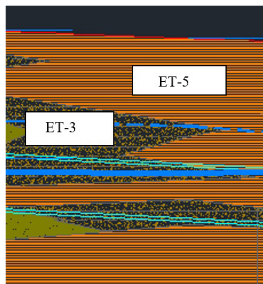
شکل (۲): پروفیل زمین شناسی محل تقاطع تونل خط ۷ با کانال رباط کریم [۱]
