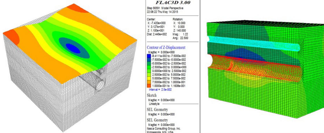
شکل (۹): تصویر مدل ساخته شده نشست ۵ سانتیمتری در سطح زمین و در مرکز مدل
