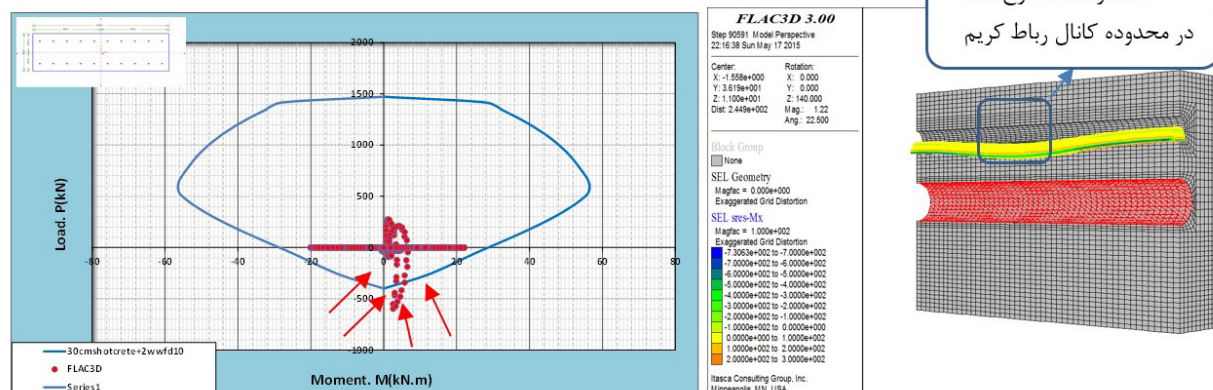
شکل (۱۱): منحنی اندرکنش سیستم نگهداری سازه کانال رباط کریم
