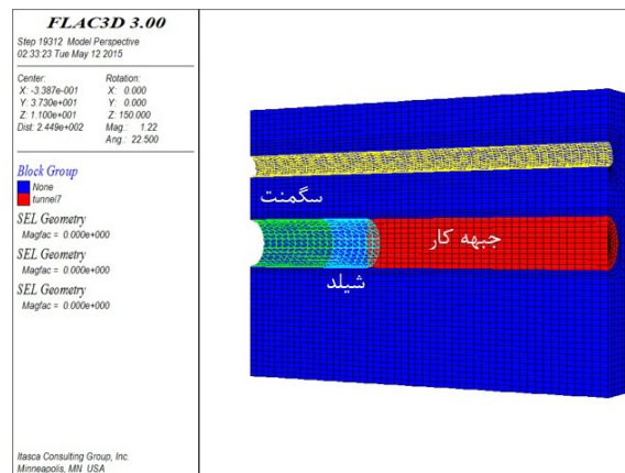
شکل (۶): سیستم نگهداری تونل خط ۷ شامل پوشش نهایی و سپر
