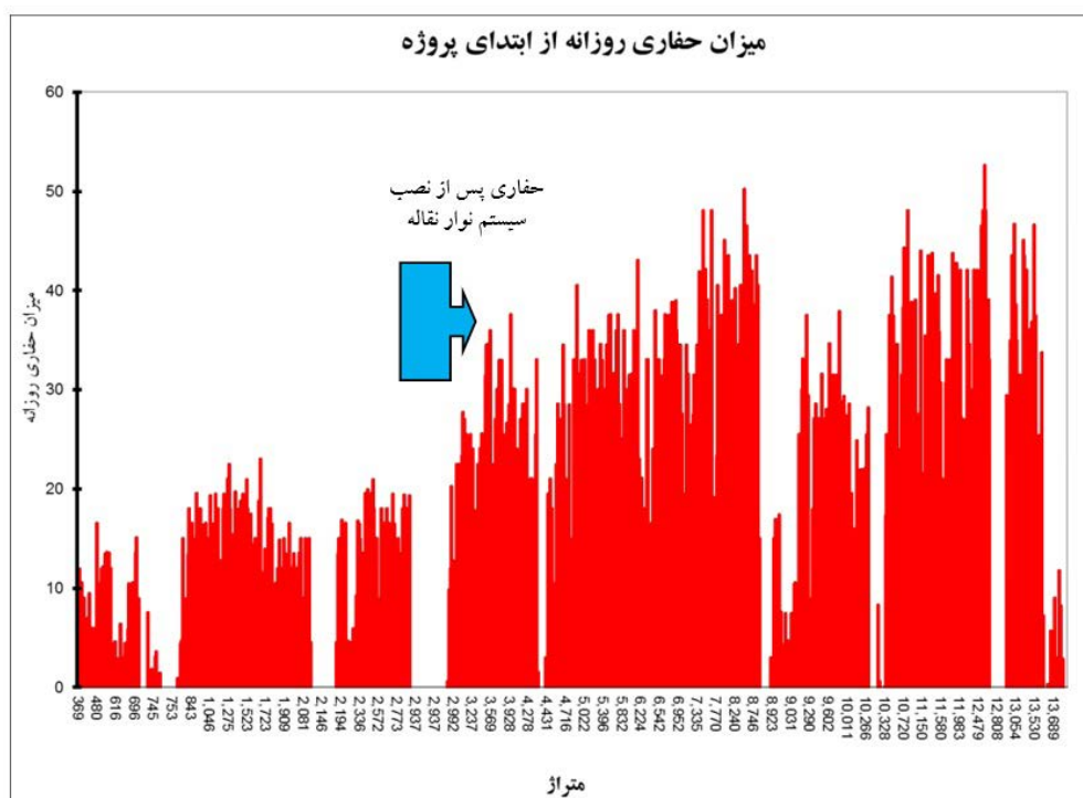
شکل (۹): میزان پیشروی روزانه بر حسب متر اژ حفاری
