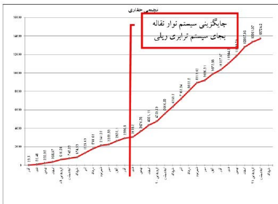
شکل (۱۰): متوسط حفاری ماهانه و میزان تجمعی حفاری در پروژه تونل بلند زاگرس
