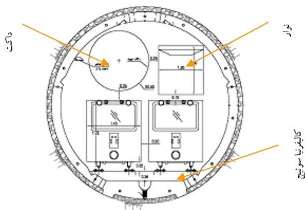
شکل (۷): جانمایی نصب نوار نقاله در تونل در محل نصب کالیفرنیا سوئیچ
