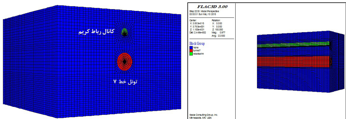
شکل (۳): هندسه مدل و ابعاد و اندازه تونل‌ها نسبت به هم با استفاده از نرم افزار FLAC3D
