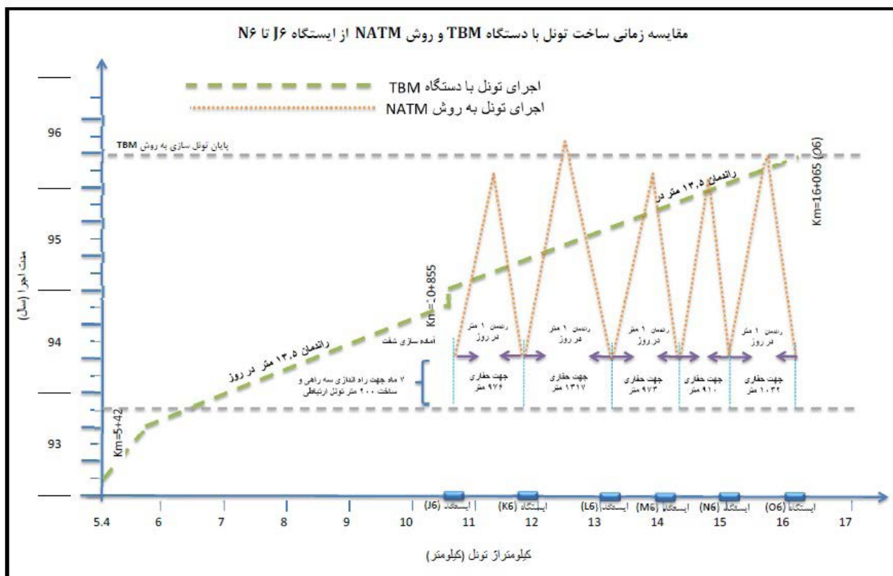
شکل ۱- مقایسه زمانی ساخت تونل با دستگاه TBM و روش NATM از ایستگاه J۶ تا N۶ خط ۶ متروی تهران
