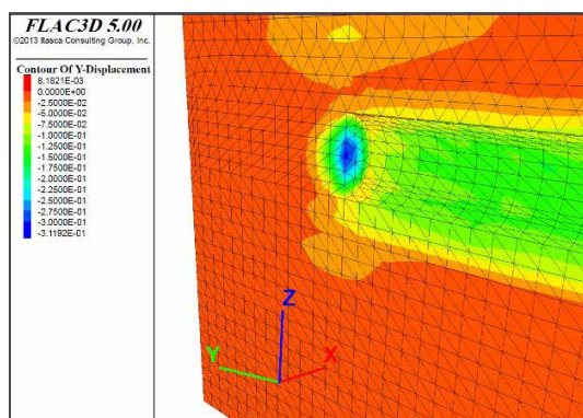
شکل ۷- کنتور جابجایی افقی در راستای محور تونل - راستای Y (واحد بر حسب متر)
