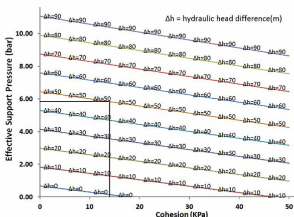
شکل ۴- رابطه بین فشار موثر مورد نیاز برای پایداری سینه کار (S) و چسبندگی (C) در (\Delta h) های مختلف
