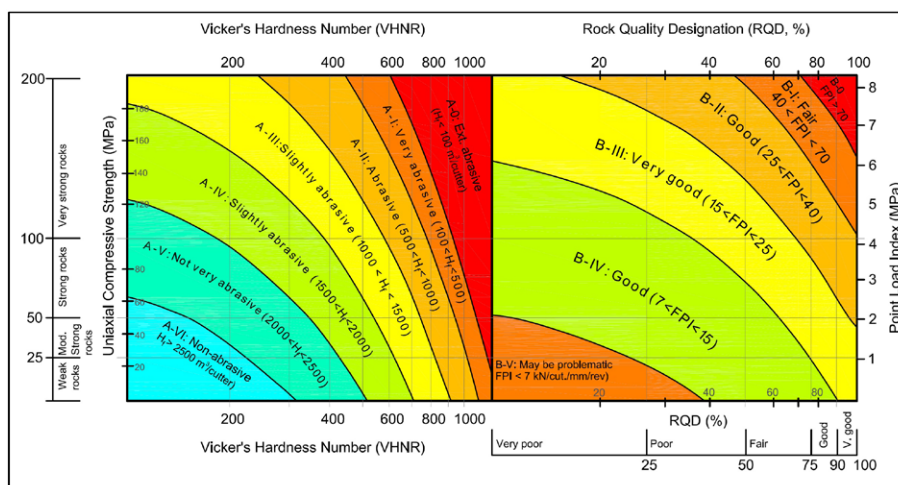
شکل ۲- مدل عمومی برای پیش‌بینی شاخص نفوذ صحرایی و عمر دیسک کاترها و رده حفریذیری و ساینده‌گی توده سنگ‌ها (حسن پور و همکاران، ۲۰۱۵)
