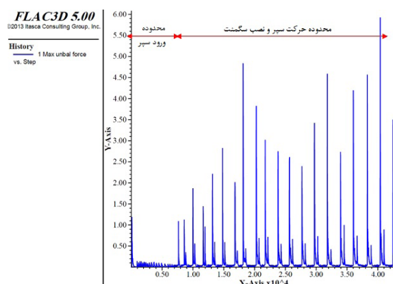
شکل ۹- تاریخچه نیروهای نامتعادل کننده مدل در سکناس های پیشروی (محور افقی سیکل محاسباتی - محور قائم ماکزیمم نیروی نامتعادل کننده بر حسب مگا نیوتن)
