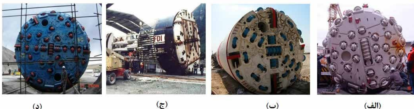
شکل ۱- نمایی از ماشین‌های حفاری در پروژه‌های الف (قمرود، ب) کرج، ج) ماناپوری و د) زاگرس
