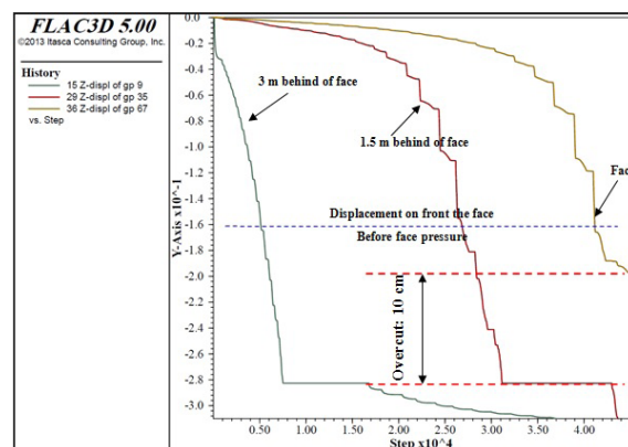
شکل ۶- تاریخچه جابجایی قائم در تاج تونل در سکناس های پیشروی (محور افقی سیکل محاسباتی - محور قائم جابجایی بر حسب متر)
