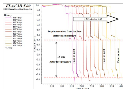
شکل ۸- تاریخچه جابجایی سینه کار در راستای افقی (محور Y) با توجه به سکناس های پیشروی (محور افقی سیکل محاسباتی - محور قائم جابجایی بر حسب متر)
