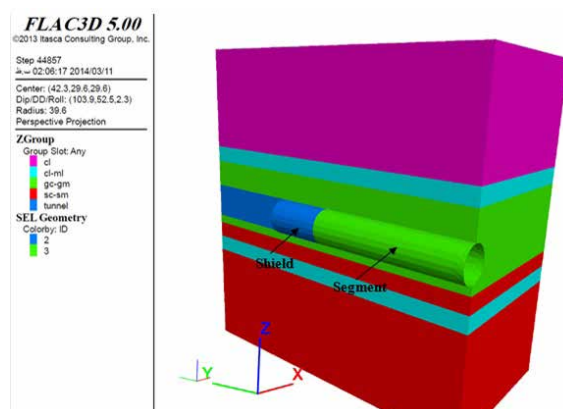
شکل ۵- المان های مدلسازی شده در نرم افزار FLAC3D
