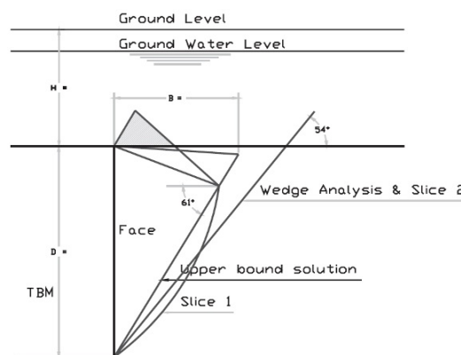
شکل ۲- سطوح بحرانی جهت آنالیز فشار سینه کار TBM [۱۴]
