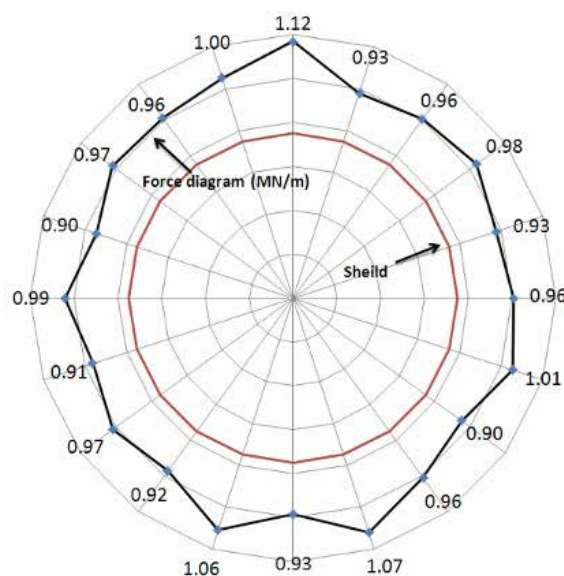
شکل ۱۱- نیروهای وارد شده در هر متر از طول سپر معادل (واحد بر حسب مگانیوتن)
