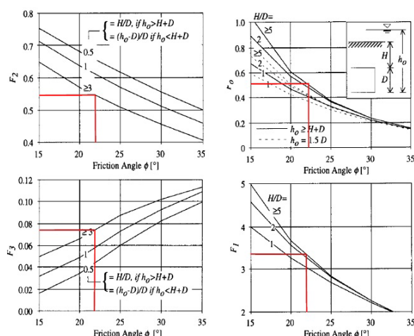
شکل ۳- ضرایب ثابت جهت تعیین فشار سینه کار [۱۵]
