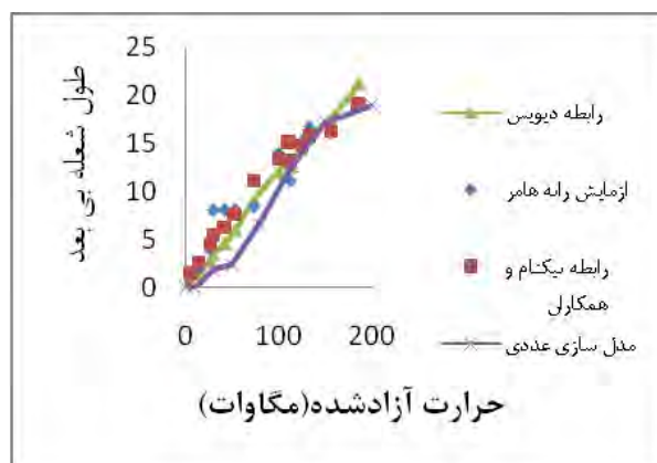
شکل ۱۰- مقایسه طول شعله آزمایش رانه هامر و فرمول ۱۳ و دیویس
