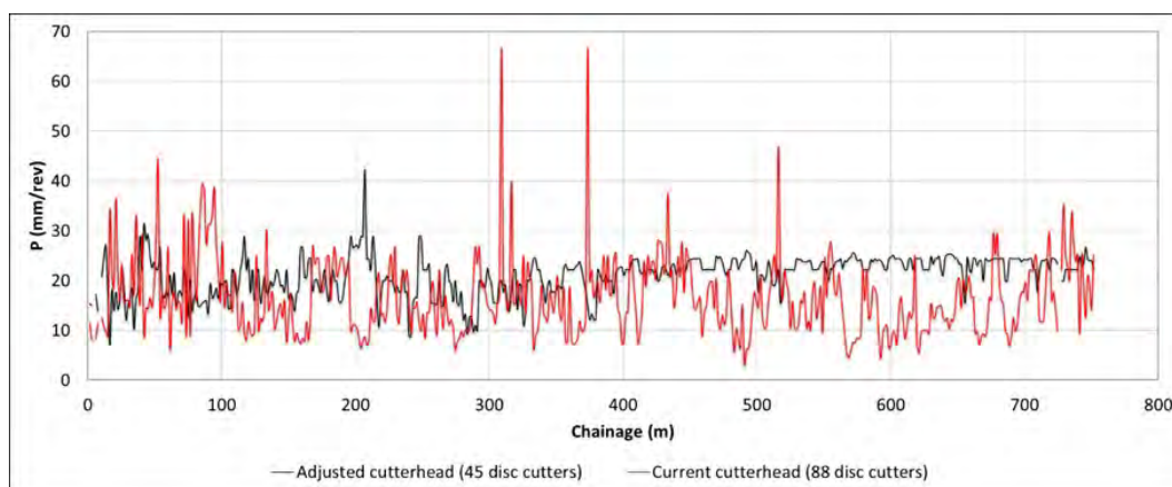
شکل ۱۲- تغییرات مقادیر نفوذ در سنگ در حالت فعلی کاترهد و با فرض نصب ۴۵ دیسک بر روی کاترهد
