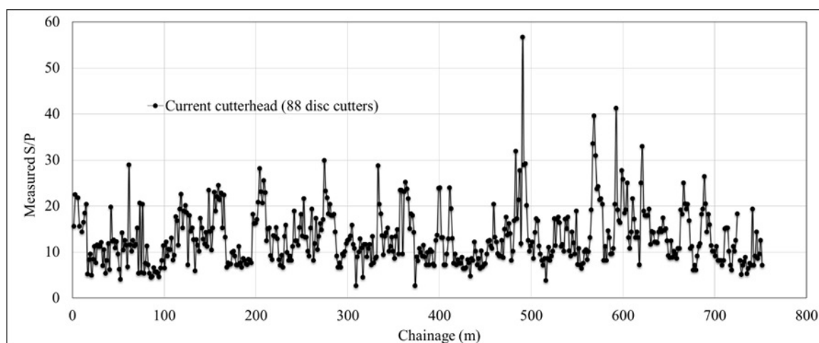
شکل ۱۰- تغییرات مقادیر نسبت S/P در مسیر حفاری شده
