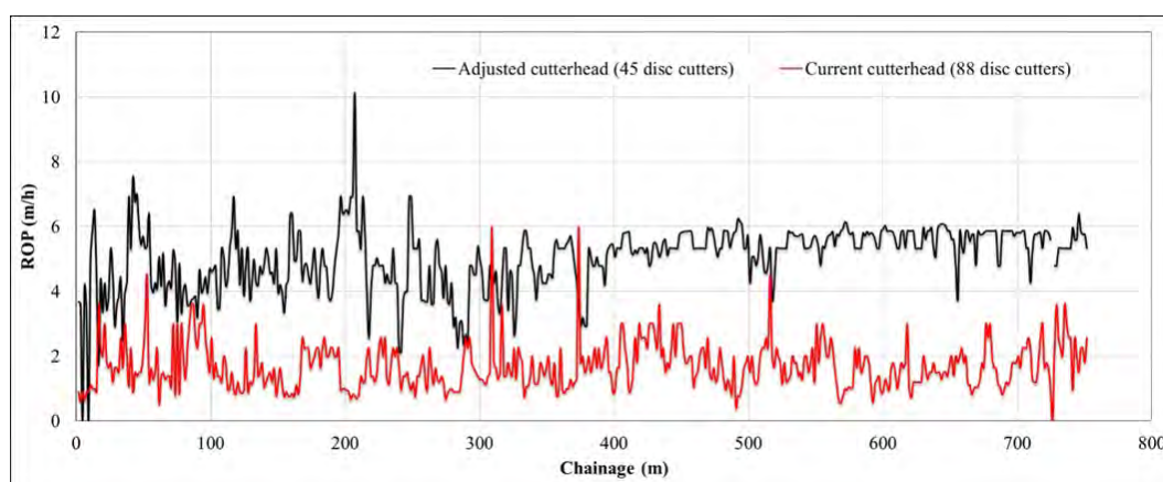
شکل ۱۵- تغییرات مقادیر نرخ نفوذ در حالت فعلی کاترهد و با فرض نصب ۴۵ دیسک بر روی کاترهد و افزایش دور دستگاه به RPM=4
