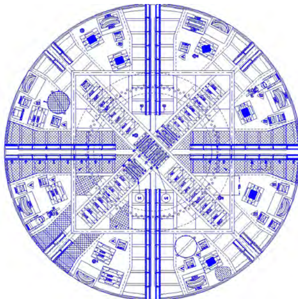
شکل ۵- نمایی از کاترهد دستگاه حفار تونل انتقال آب بازی دراز
