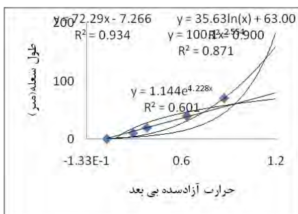
شکل ۲- تعیین بهترین رابطه برای بیان ارتباط بین حرارت آزاد شده و طول شعله آتش در آزمایش شماره T_1 تونل رانه هامر
