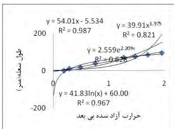
شکل ۳- تعیین بهترین رابطه برای بیان ارتباط بین حرارت آزاد شده و طول شعله آتش در آزمایش شماره T_2 تونل رانه هامر
