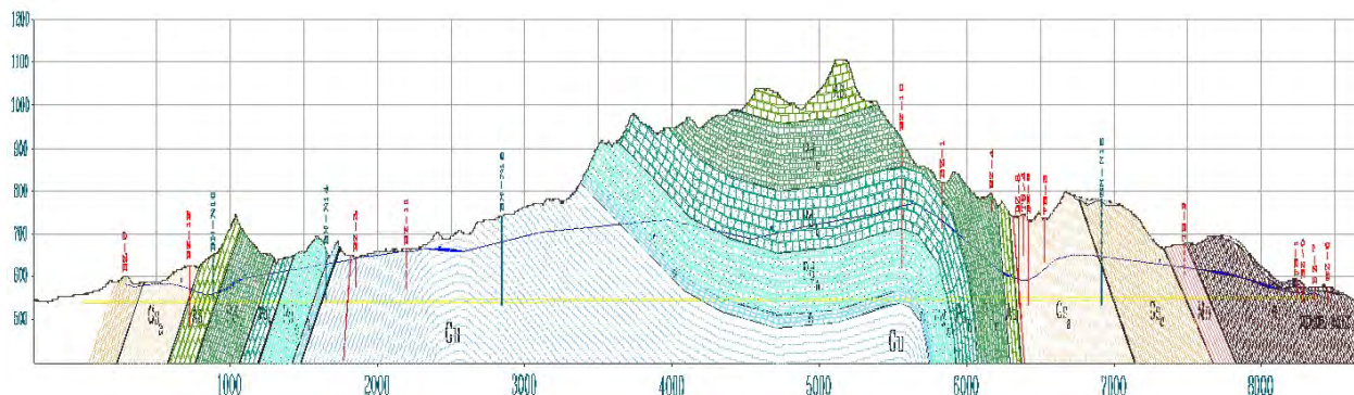
شکل ۱- پروفیل زمین شناسی مسیر تونل بازی دراز
