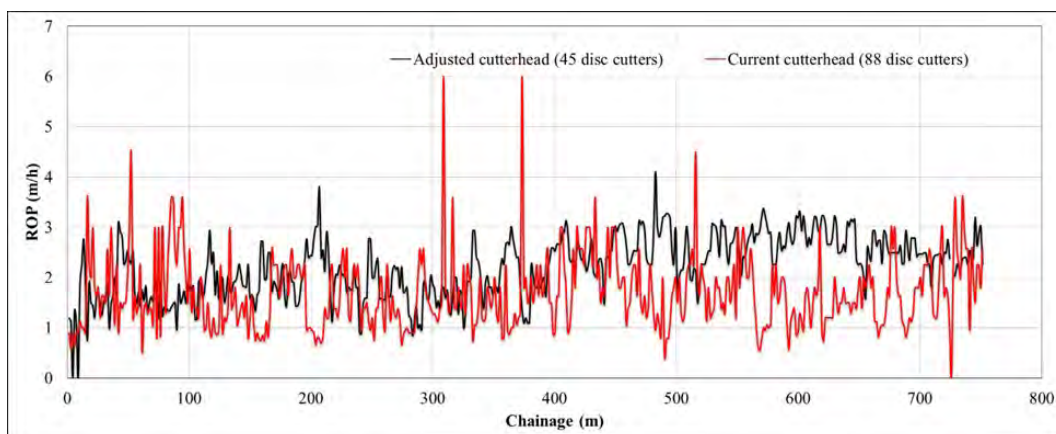
شکل ۱۳- تغییرات مقادیر نرخ نفوذ در حالت فعلی کاترهد و با فرض نصب ۴۵ دیسک بر روی کاترهد
