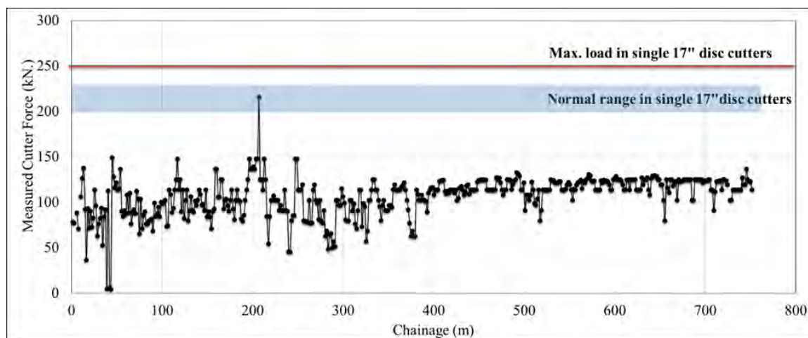
شکل ۸- تغییرات مقادیر متوسط نیروی اعمالی به هر دیسک Fn در مسیر حفاری شده
