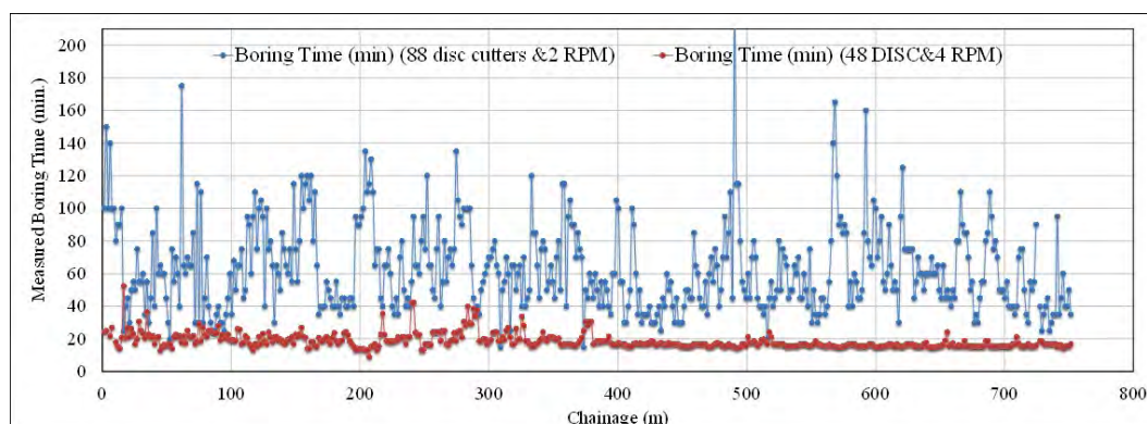
شکل ۱۶- تغییرات مقادیر زمان حفاری با فرض نصب ۴۵ دیسک بر روی کاترهد و افزایش دور دستگاه به RPM=4
