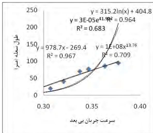
شکل ۴- تعیین بهترین رابطه برای بیان ارتباط بین سرعت جریان و طول شعله آتش در آزمایش شماره T 3 تونل رانه هامر
