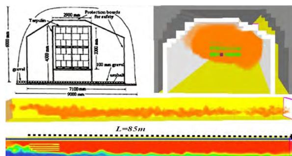
شکل ۹- هندسه تونل رانه هامر مدل ساخته شده و طول شعله در لحظه حداکثر آتش سوزی
