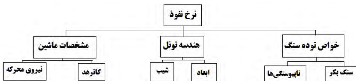
شکل ۴- پارامترهای مؤثر در نرخ نفوذ TBM
