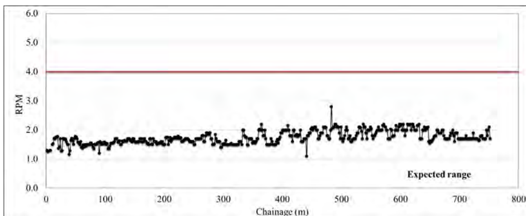
شکل ۱۴- تغییرات RPM یا دور دستگاه در بخش حفاری شده
