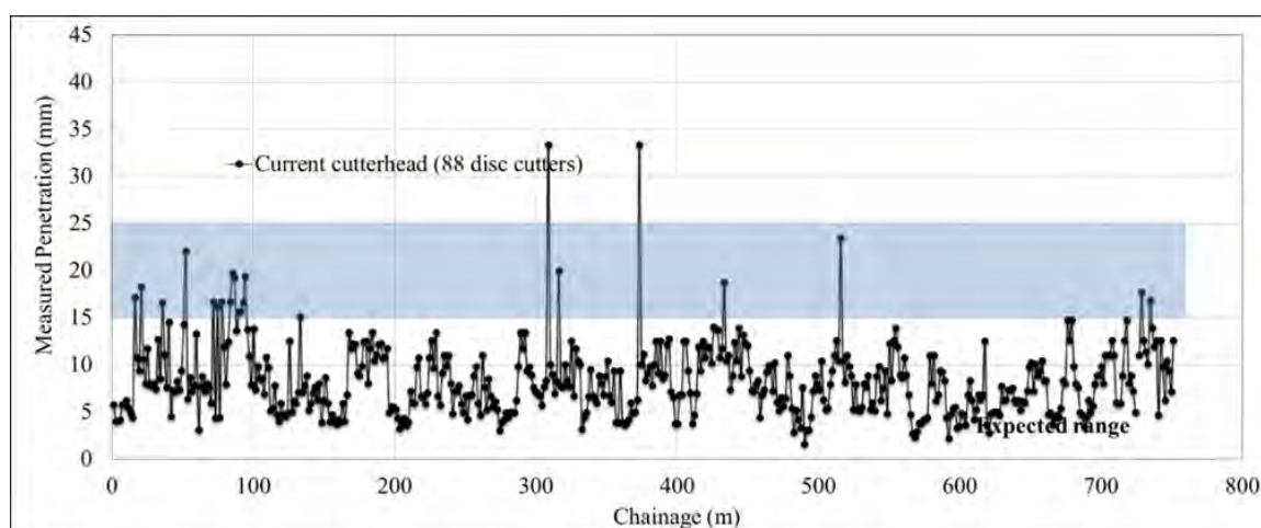
شکل ۹- تغییرات مقادیر نفوذ دیسک یا P در مسیر حفاری شده
