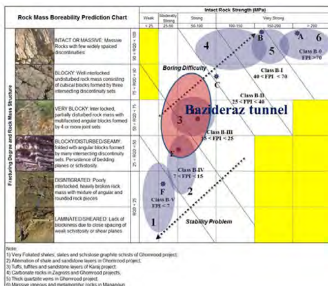
شکل ۳- مدل عمومی برای پیش بینی شاخص نفوذ صحرایی و رده حفریذری توده سنگ
