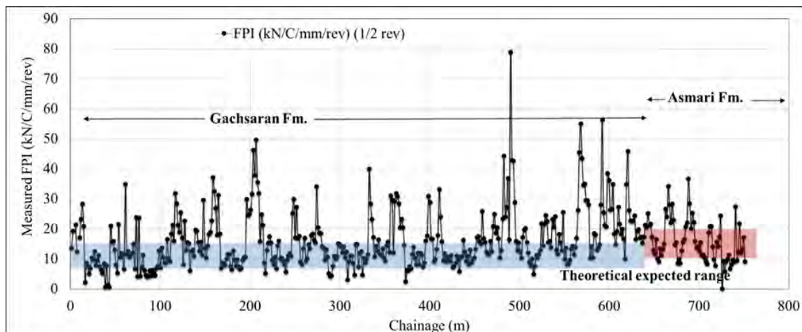
شکل ۶- دامنه تغییرات پارامتر FPI و مقایسه آن با مقادیر مورد انتظار
