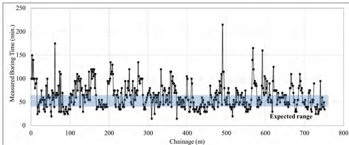
شکل ۷- تغییرات مقادیر زمان خالص حفاری یک کورس در مسیر حفاری شده
