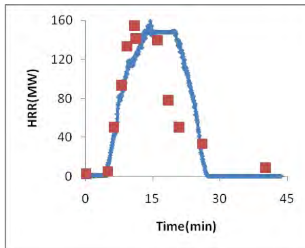
شکل ۸- حرارت آزاد شده از مدل ساخته شده و آزمایش تونل رانه هامر
