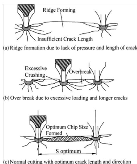
شکل ۲- مکانیسم برش در سنگ با توجه به فاصله دیسک ها و میزان نفوذ و نیروی قائم اعمال شده به سینه کار از سوی دیسک ها
