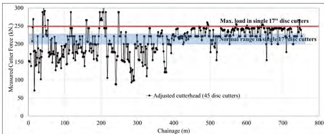
شکل ۱۱- تغییرات مقادیر متوسط نیروی اعمالی به هر دیسک F_n با فرض نصب ۴۵ دیسک بر روی کاترهد
