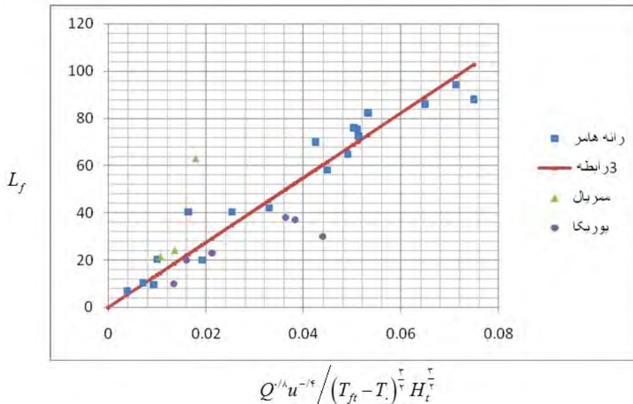
شکل ۱- مقایسه طول شعله حاصل از رابطه ۳ با آزمایش های بزرگ مقیاس آتش سوزی
