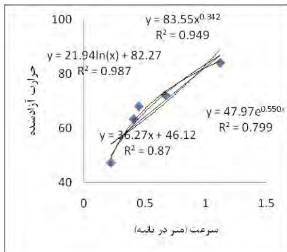
شکل ۵- تعیین بهترین رابطه برای بیان ارتباط بین سرعت جریان و طول شعله آتش در آزمایش شماره T 3 تونل رانه هامر
