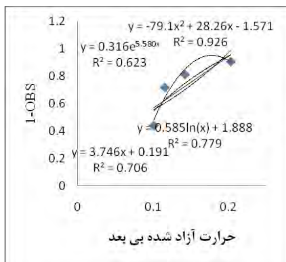
شکل ۷- تعیین بهترین رابطه برای بیان ارتباط بین انسداد تونل و حرارت آزاد شده مدل سرکان کاپلی
